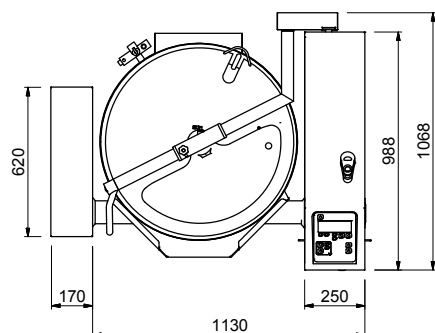
Boven aanzicht
